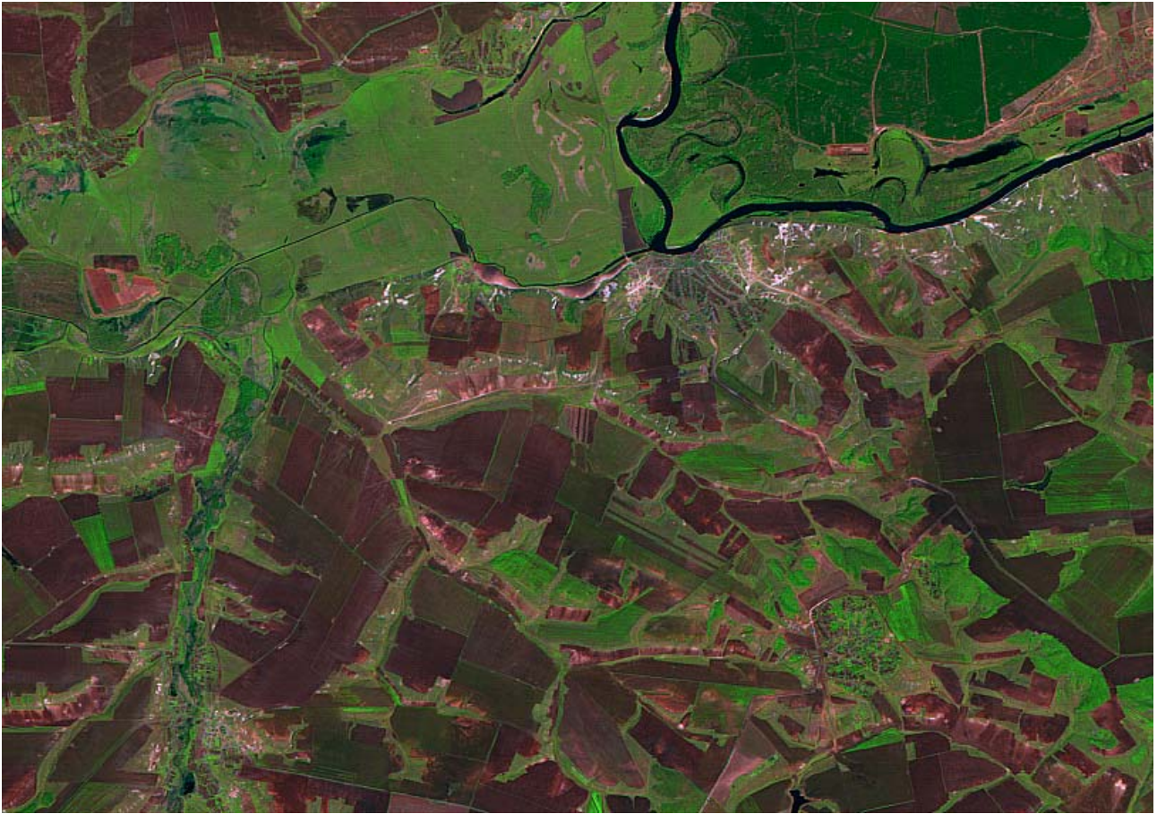
Figura 1 – Particolare del fotomosaico ottenuto dalla composizione in falso colore delle bande TM 5, 4 e 3 relativo all'area del "quadrivio di Selenyj Jar"
