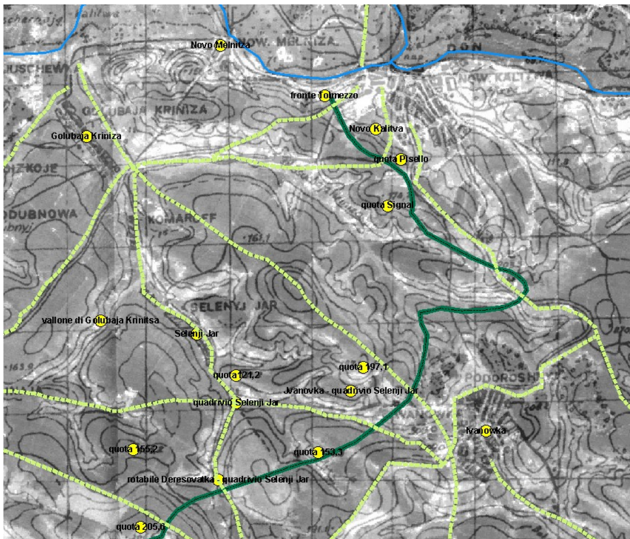
Figura 3 – Esempio di sovrapposizione di dati telerilevati, cartografici e tematici relativi all'area del “quadrivio di Selenyj Jar”. I toponimi sono stati identificati per la loro rilevanza storica, derivata dai testi consultati.
