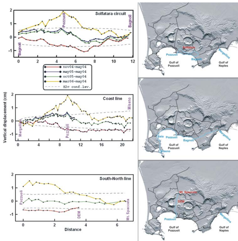
Fig. 2: Variazioni di quota nel periodo maggio 2004-Marzo 2006 lungo il Circuito Solfatara, la linea costiera e la linea Sud -Nord. Le linee tratteggiate delimitano i livelli di confidenza \pm 2\sigma .
