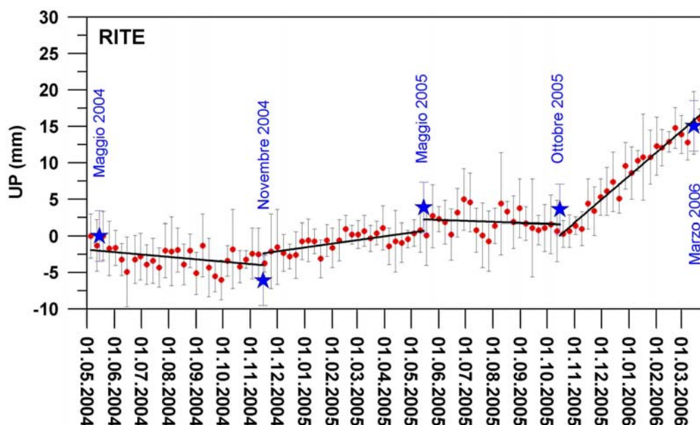
Fig. 4: Serie temporale (maggio 2004 – marzo 2006) delle variazioni settimanali in quota della stazione CGPS di RITE (Rione Terra - Pozzuoli). Sono riportate anche le curve di regressione lineare per i quattro intervalli temporali considerati. Le stelle blu indicano le variazioni di quota calcolate dalle campagne di livellazione effettuate nel 2004, 2005 e 2006, rispetto a maggio 2004 per il caposaldo più prossimo alla stazione CGPS.
