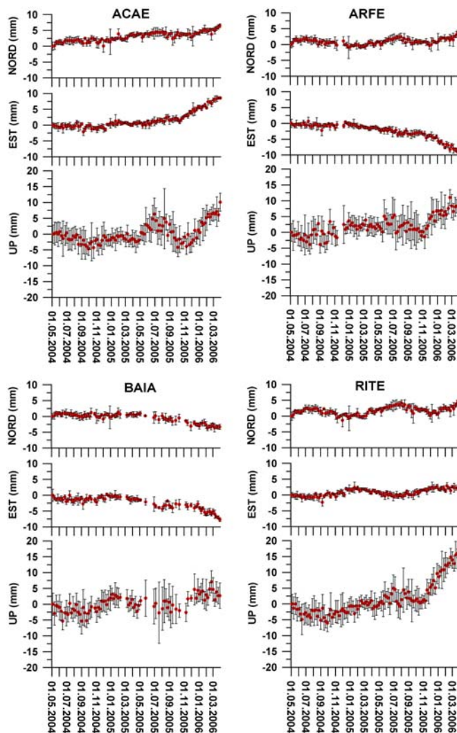
Fig. 3: Serie temporali (maggio 2004 – marzo 2006) delle variazioni settimanali in Nord, Est ed Up delle coordinate delle stazioni CGPS di ACAE, ARFE, BAIA e RITE relativamente a QUAR. Elaborazione effettuata con il software Bernese v. 4.2.
