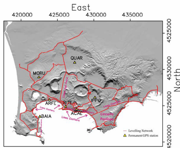
Fig. 1: Rete altimetrica dei Campi Flegrei. Sono riportate con triangoli gialli le stazioni CGPS.
