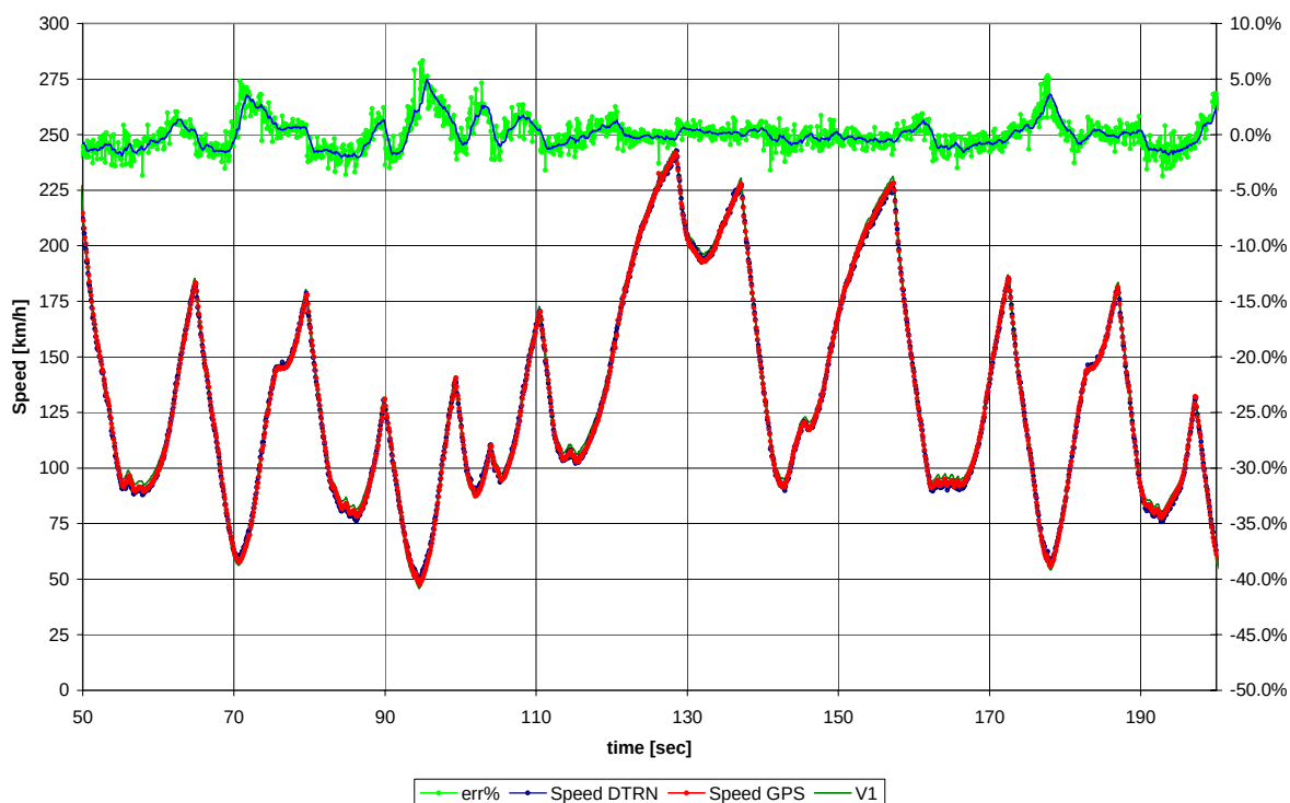
Figura 6 – sovrapposizione dei profili di velocità acquisiti con il sensore ottico (speed DTRN), con la ruota fonica (V1) e calcolati sulla base della misura GPS
